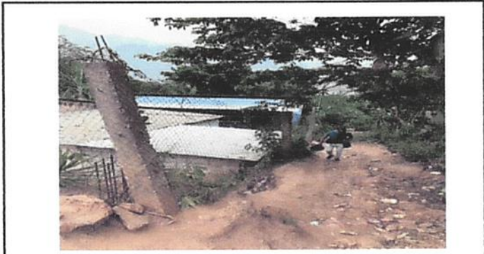
Foto 1: Muro perimetral 5 hiladas de block con tubo galvanizado para cerca de 1 1/2" y malla galvanizada de 1.50 mts de alto con alambre de púa.
